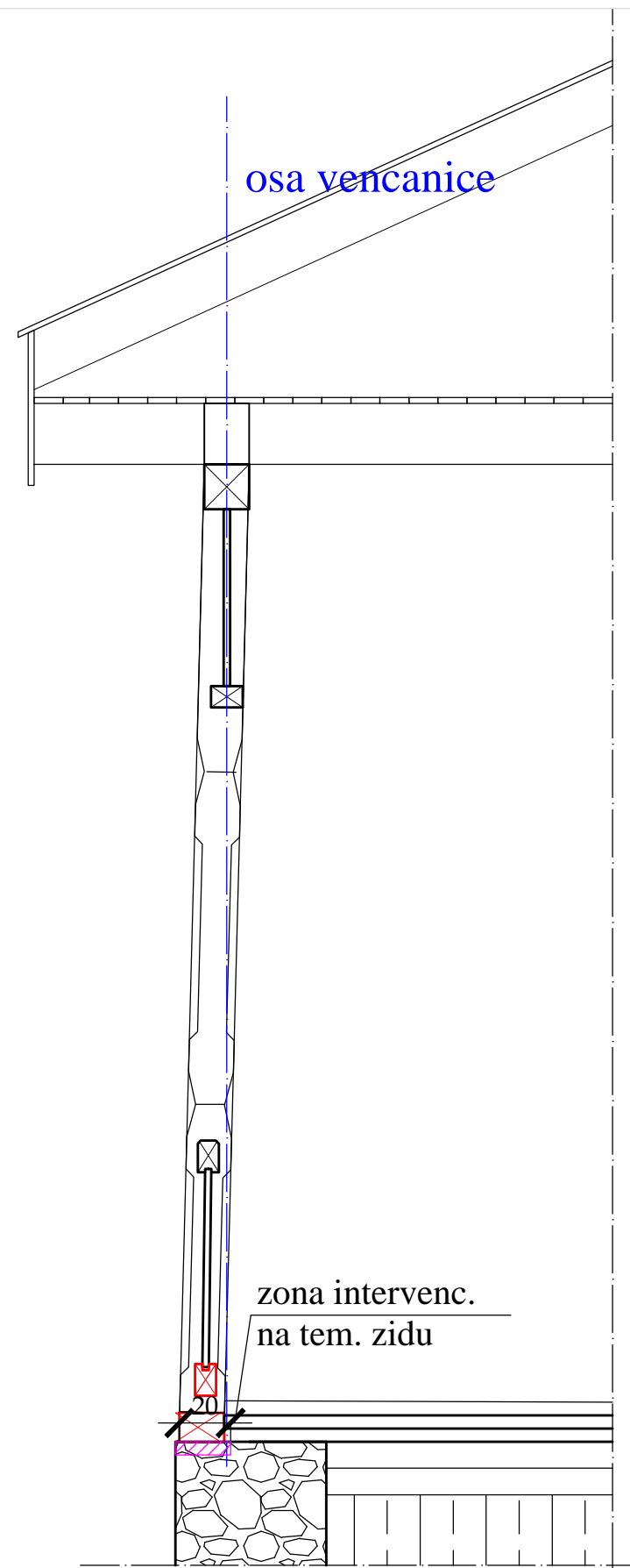
PRESEK 1-1
