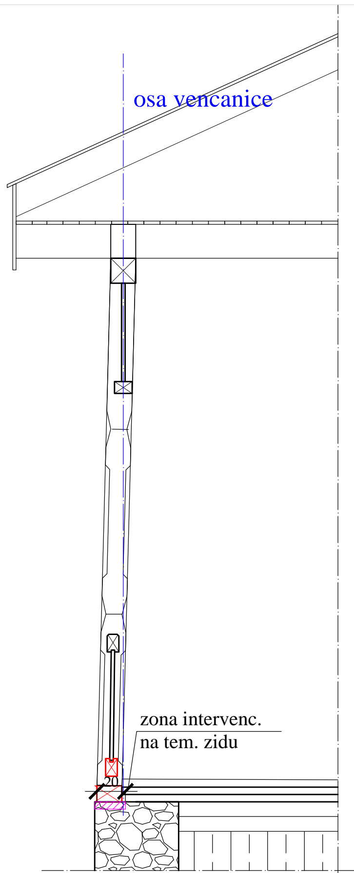
PRESEK 1-1
