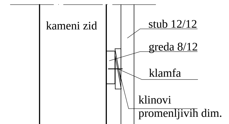
Detalj B-B učvršćivanje stubova za kamene zidove
