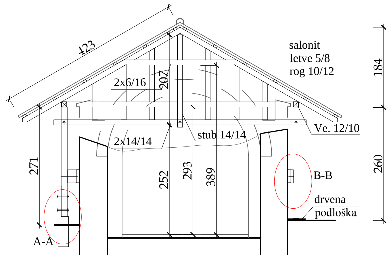
Presek 1-1
