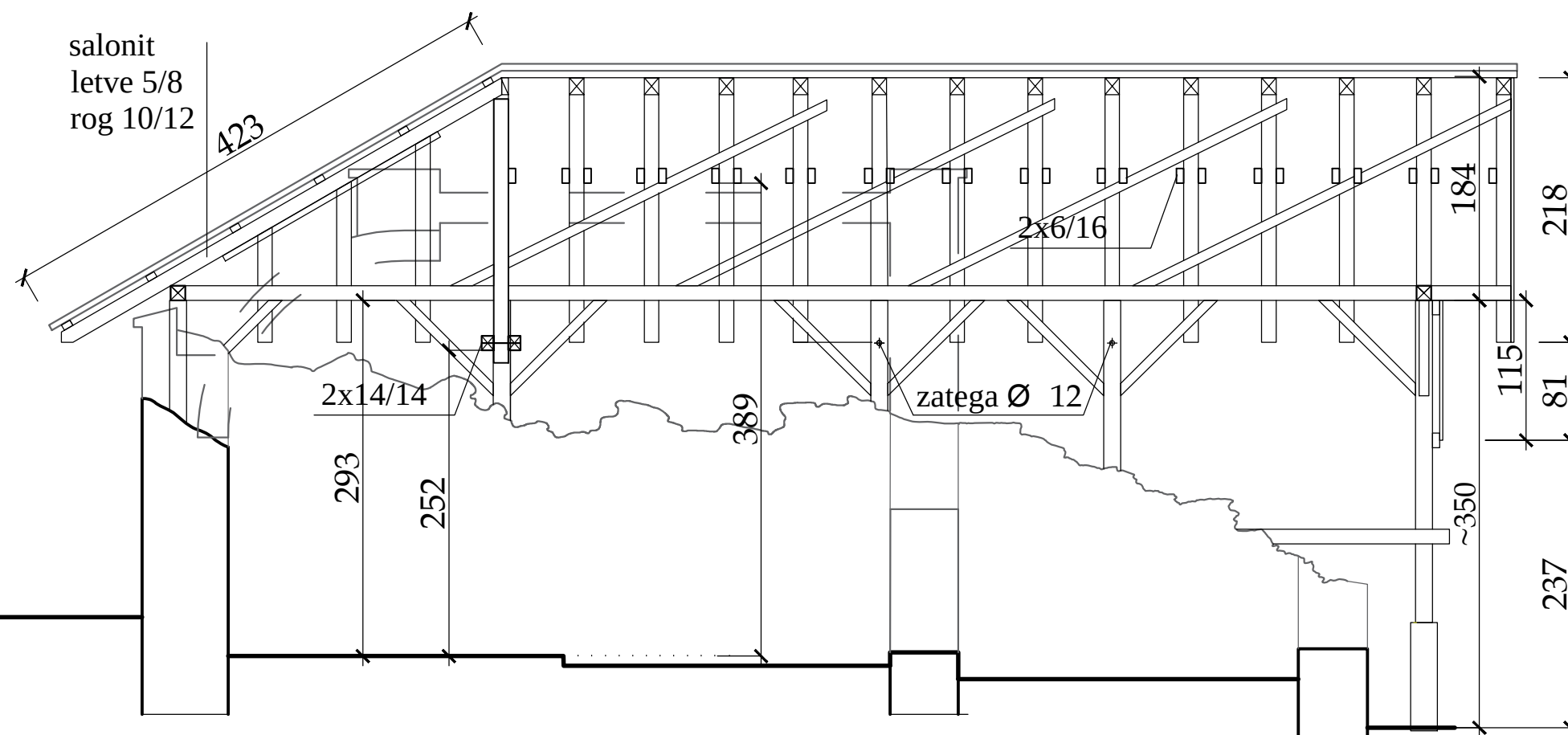
Presek 2-2
