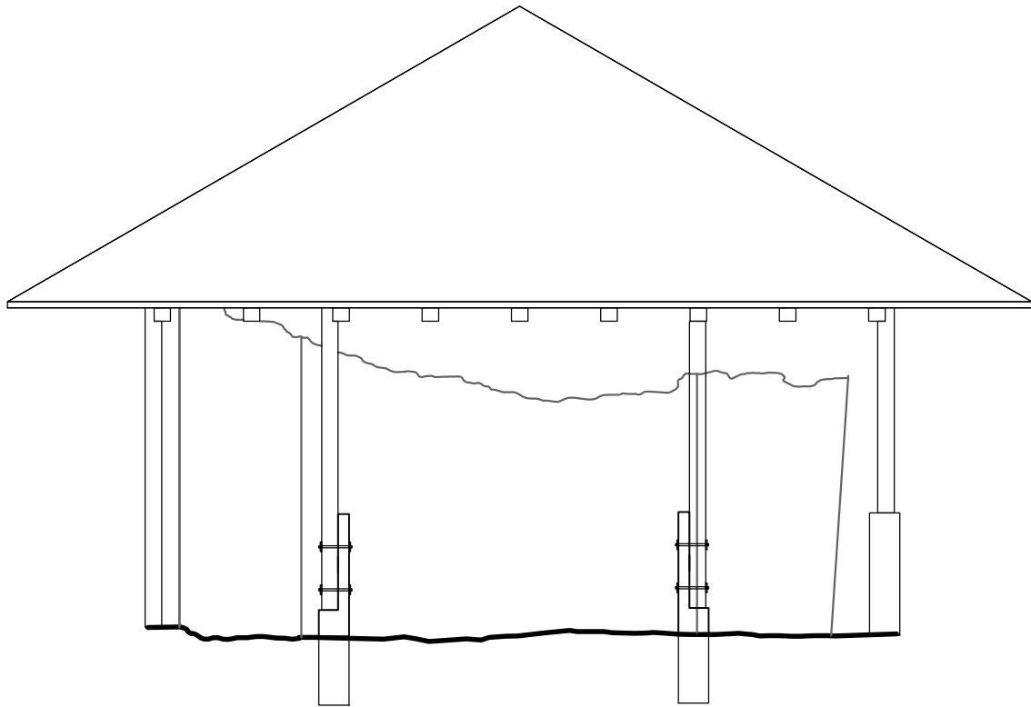
IZGLED ISTOČNI
