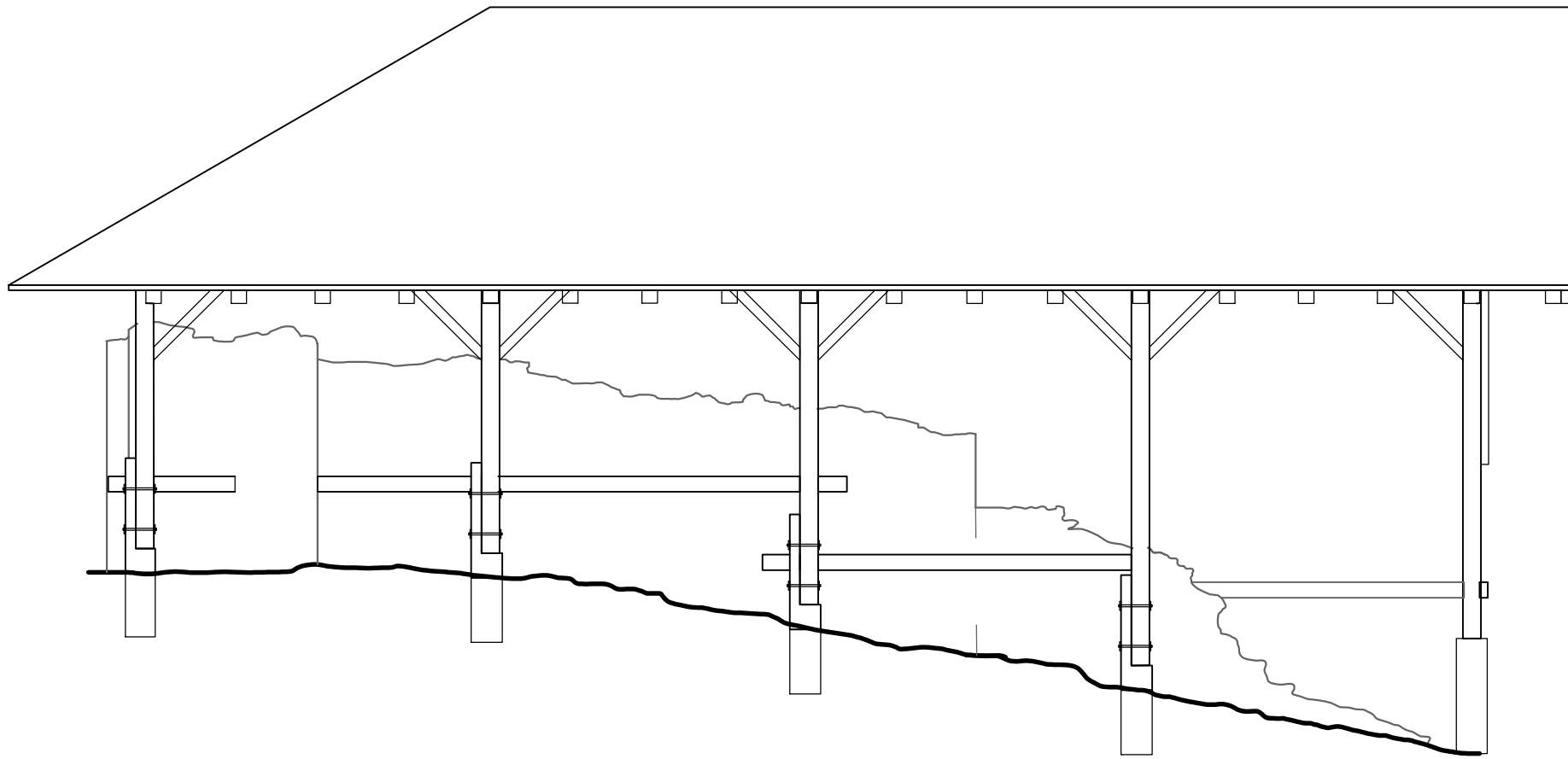
IZGLED BOČNI-SEVERNI
