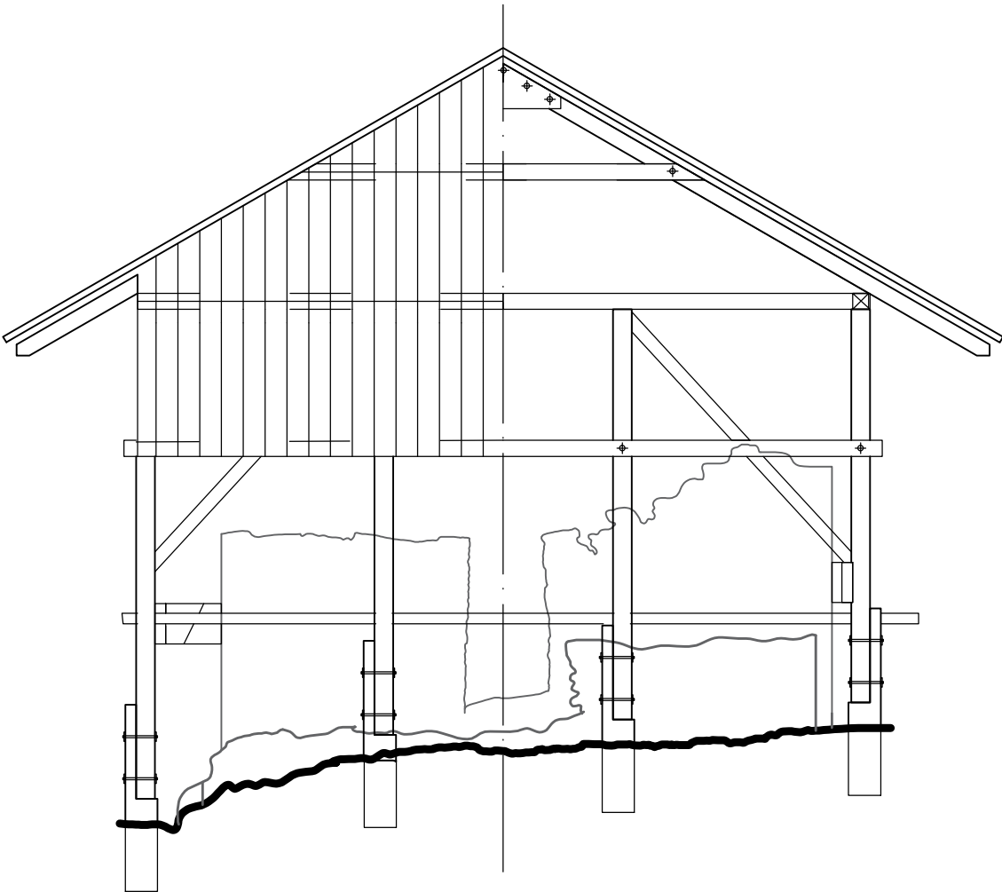
IZGLED ZAPADNI sa delimičnim izgledom konstrukcije
