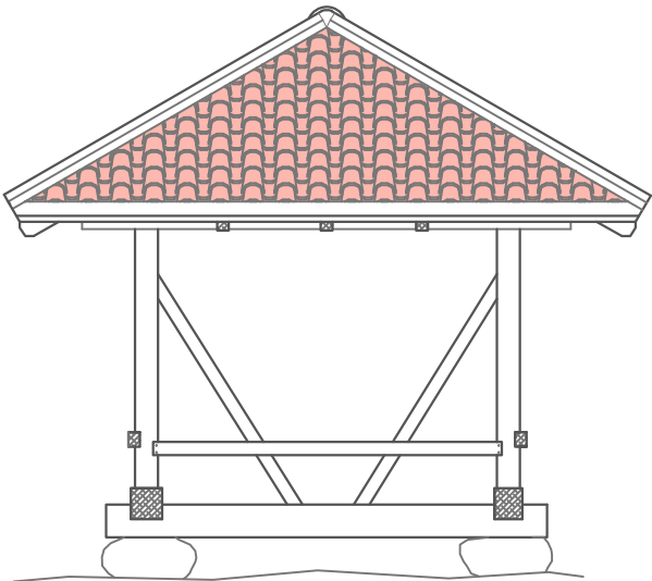
попечни изглед
