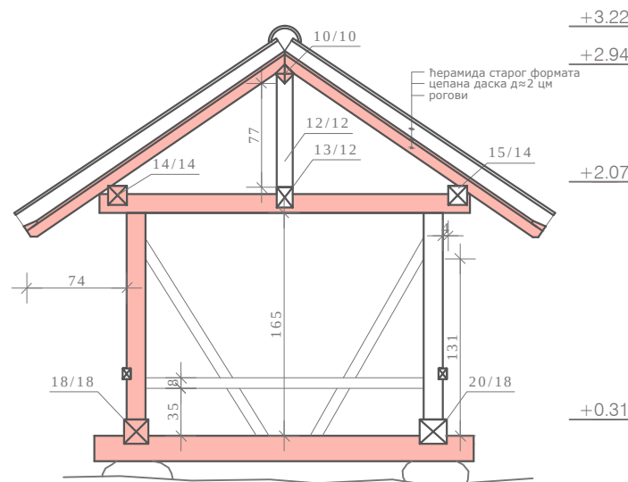
попечни пресек
