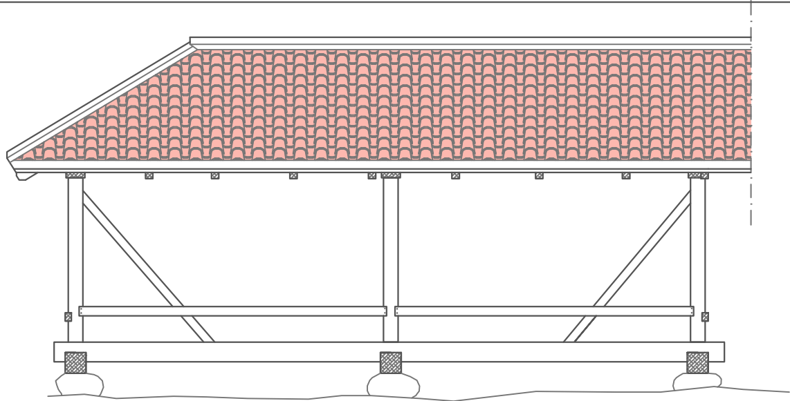
подужни изглед
