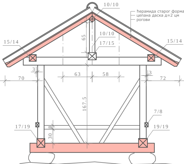
попечни пресек
