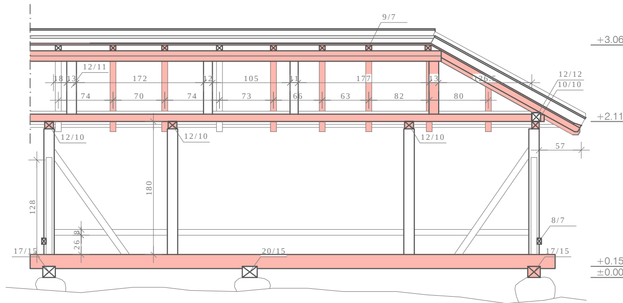
подужни пресек
