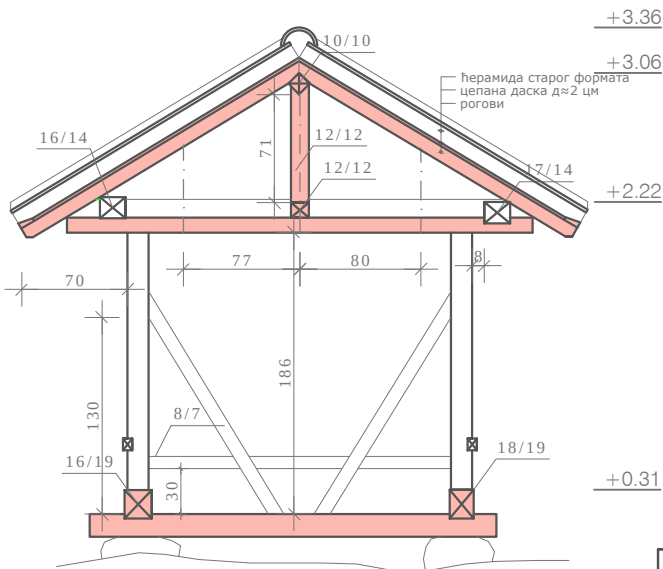
попечни пресек
