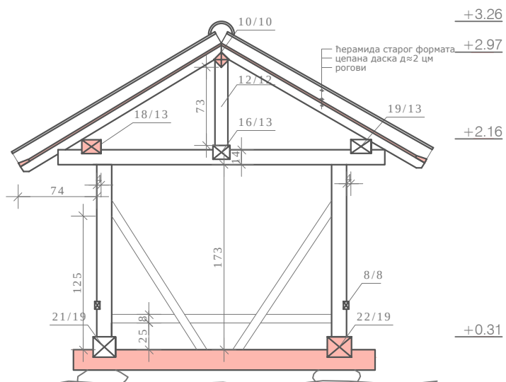
попечни пресек
