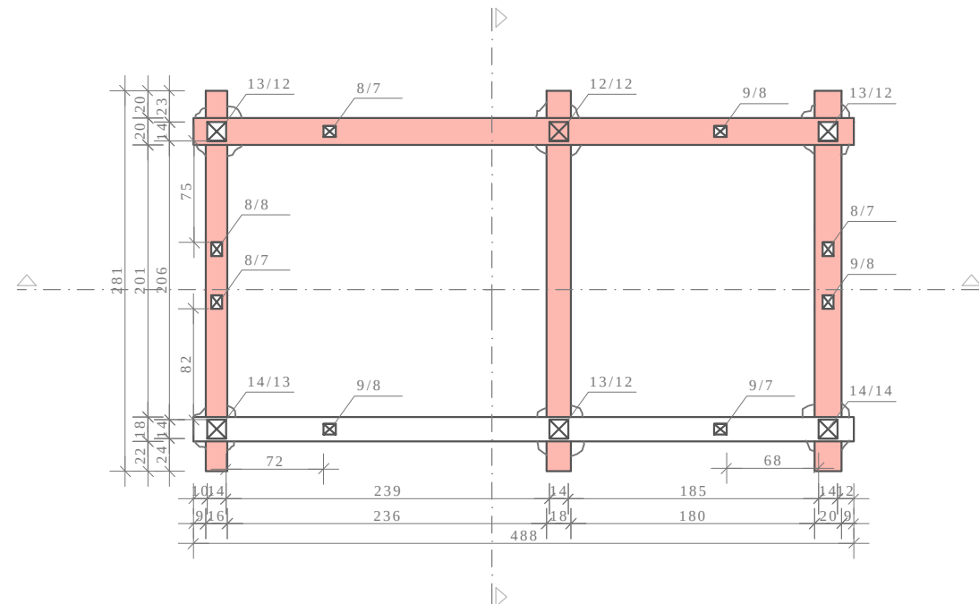
ОСНОВА
