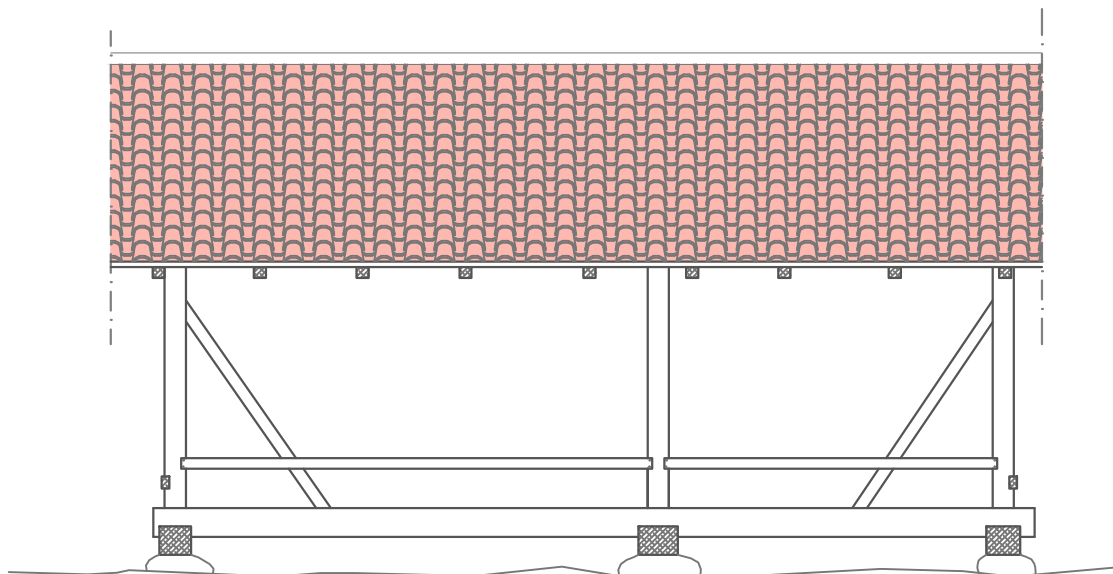
подужни изглед
