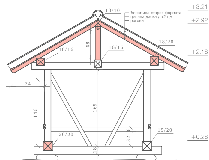
попечни пресек
