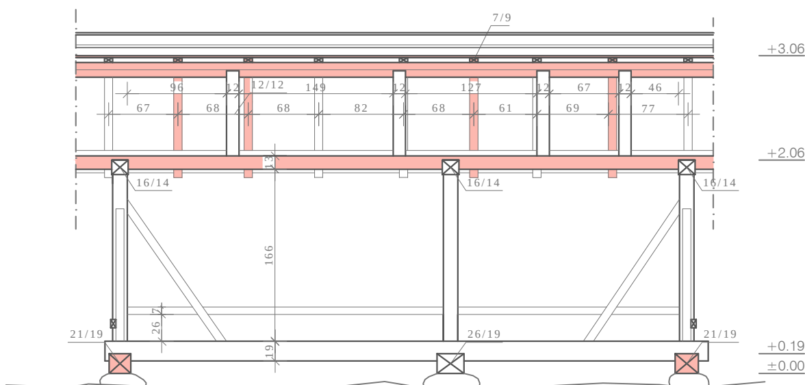
подужни пресек
