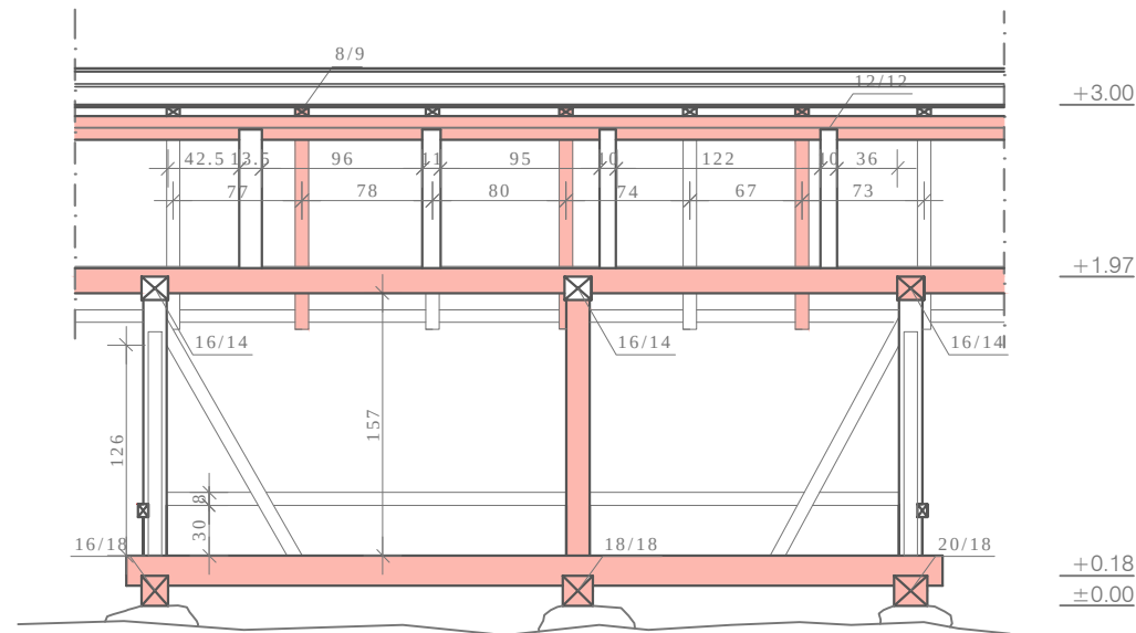
подужни изглед
