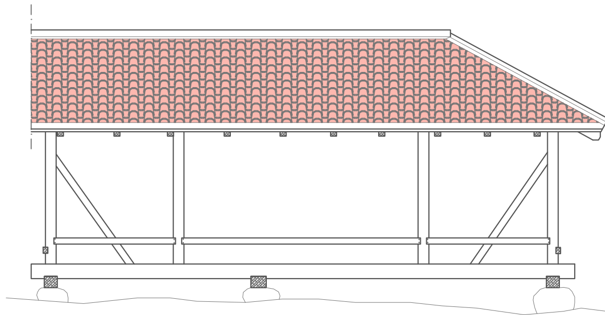
подужни изглед
